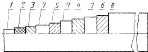
СХЕМА РУКАВА
