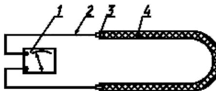
1 — измерительный прибор; 2 — проводник; 3 — электрод; 4 — рукав
